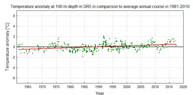
Ytvattnets temperatur i södra Bottenviken jämfört med det dagliga medelvärdet åren 1981–2010
